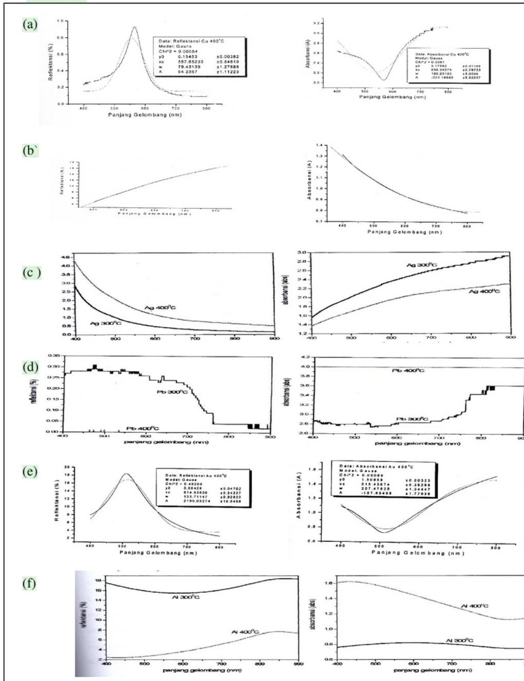
Gambar 2. Respon spektral Reflektansi dan Absorbansi Lapisan tipis pada panjang gelombang daerah UV-VIS : (a).Cu; (b). In; (c). Ag; (d).Pb; (e). Au; (f).Al
